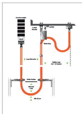
Балансировочная Цепь
